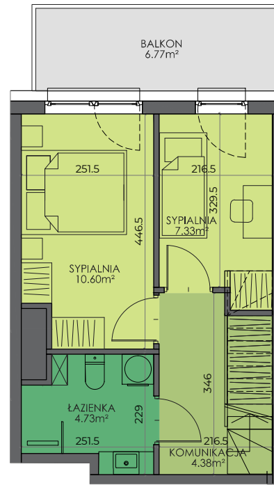
POZIOM 2 - KONDYGNACJA 7
